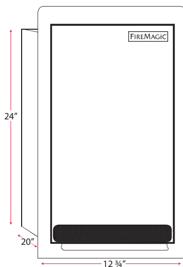
Fig. 1-1 Cutout dimensions
