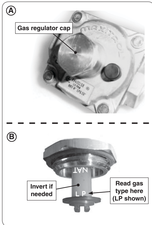
Fig. 25-1 Convert regulator
